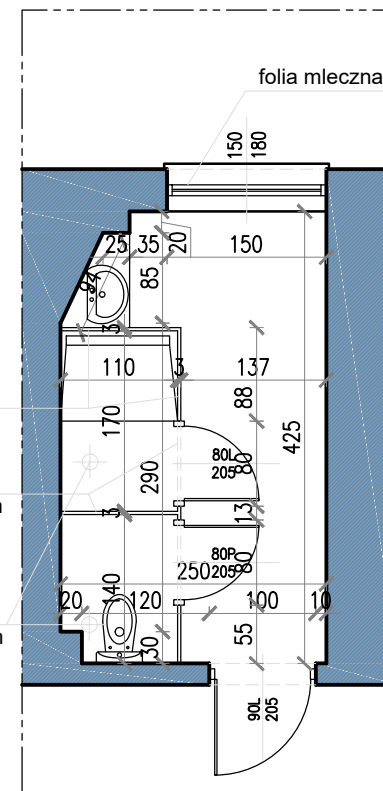
ŁAZIENKA_2- stan projektowany
