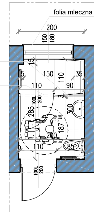
ŁAZIENKA_3- stan projektowany
