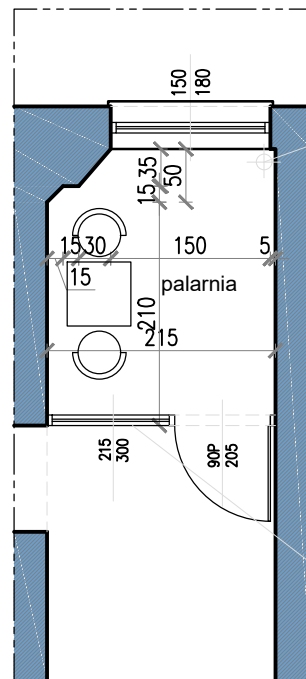
KORYTARZ-stan projektowany
