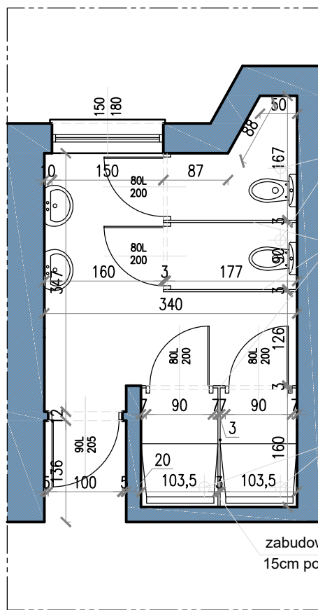
ŁAZIENKA_1- stan projektowany
