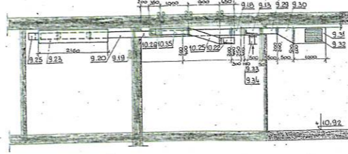
E-E 1:50
