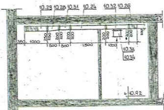
C-C 1:50
