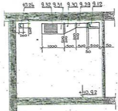
D-D 1:50
