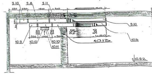
G-G 1:50
