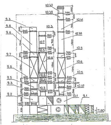
B-B 1:50
