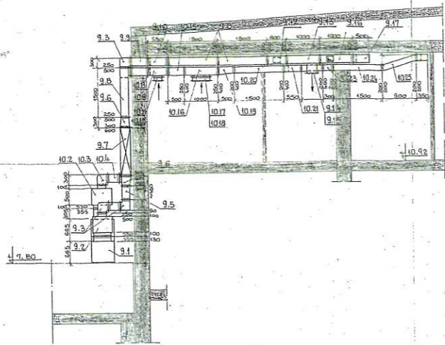
A-A 1:50
