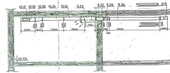
G-G 1:50
